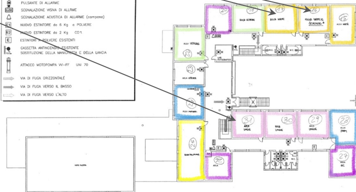
LOCALIZZAZIONE DISPOSITIVI ANTINCENDIO E VIE DI FUGA PIANO PRIMO
